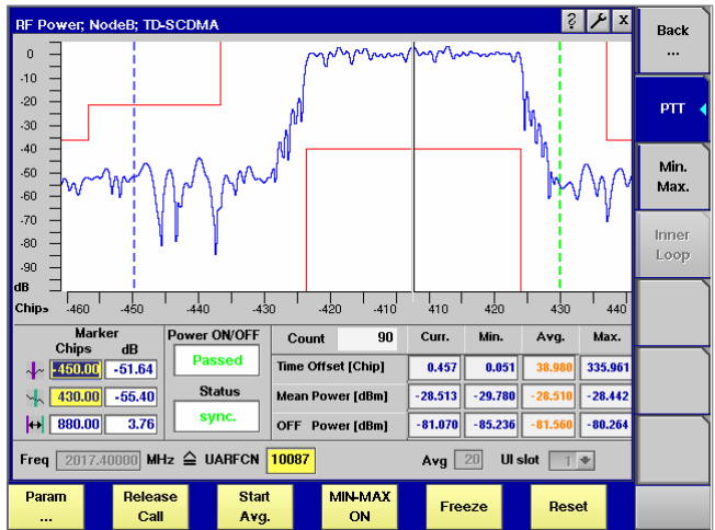
图 6：TD-SCDMA功率测量
