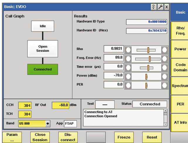
图 10：EV-DO呼叫状态图基本菜单
