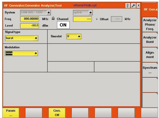
图 13：射频信号发生器/分析仪模式
