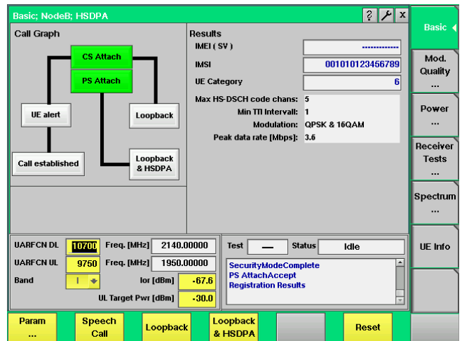
图 4： HSDPA基本连接菜单
