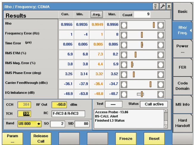
图 9：调制质量测试
