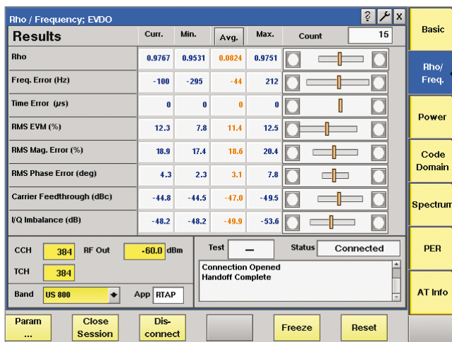
图 11：发射器质量参数概览
