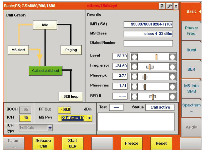
图 12：GSM基本测试屏幕显示
