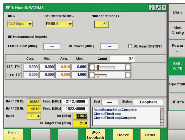
图 5：利用BER/BLER测量估算接收器灵敏度
