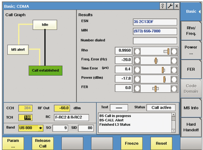
图 8：基本屏幕CDMA2000
